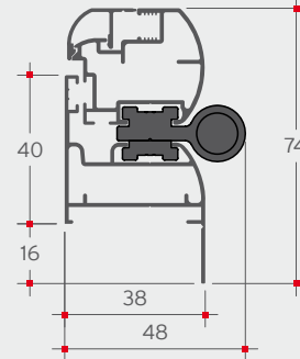
Telaio a L + compensatore + cerniera
