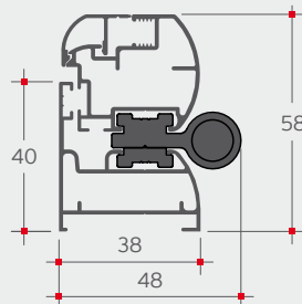
Telaio a L + cerniera
