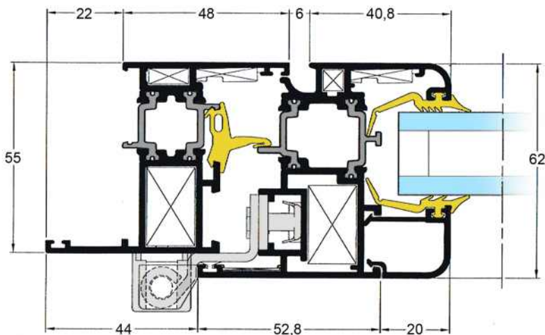
Apertura a battente
