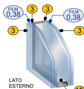
Vetro antinfortunistico (6/7 - 15 - 6/7 mm) basso emissivo
